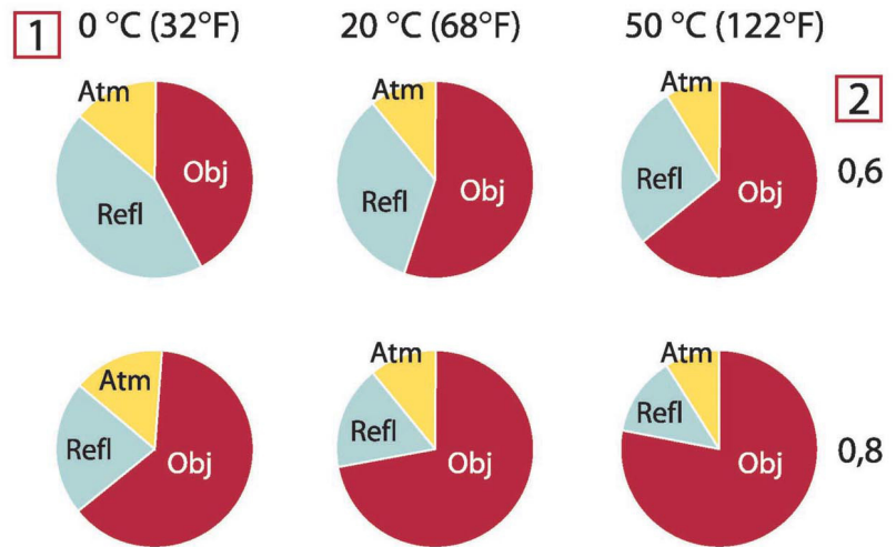
Figure 20.3 Magnitudes relatives de sources de rayonnement sous différentes conditions de mesure (caméra LW). 1 : Température de l'objet ; 2 : Exitance ; Obj : Rayonnement d'objet ; Refl : Rayonnement réfléchi ; Atm : rayonnement de l'atmosphère. Paramètres fixes : \tau = 0,88 ; T_{refl} = 20 \text{ °C} ; T_{atm} = 20 \text{ °C} .
