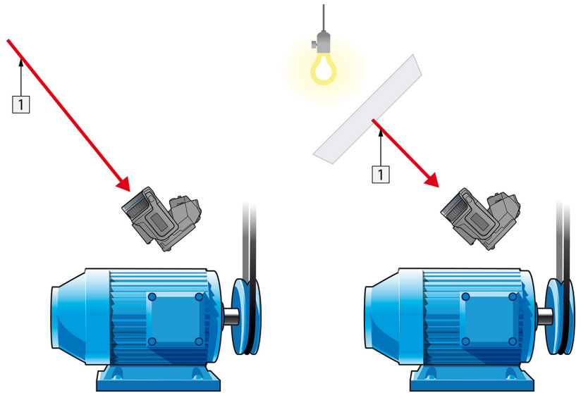
Figure 16.3 1 = Source de réflexion
