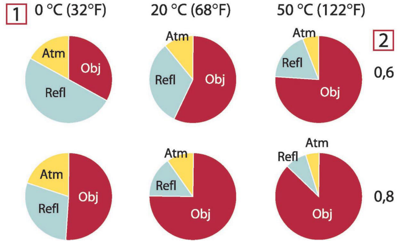
Figure 20.2 Magnitudes relatives de sources de rayonnement sous différentes conditions de mesure (caméra SW). 1 : Température de l'objet ; 2 : Exitance ; Obj : Rayonnement d'objet ; Refl : Rayonnement réfléchi ; Atm : rayonnement de l'atmosphère. Paramètres fixes : \tau = 0,88 ; T_{refl} = 20 \text{ °C} ; T_{atm} = 20 \text{ °C} .
